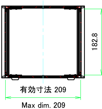
A-A ( 1 : 6 )
