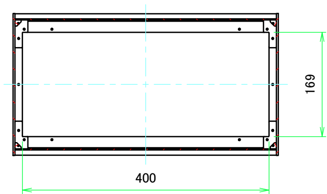
B-B ( 1 : 6 )
